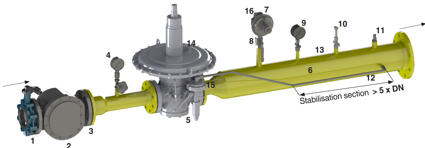
Esquema de montaje
