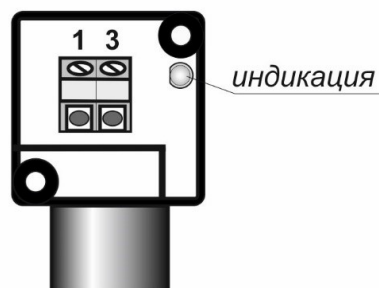
Цоколевка клеммной колодки
