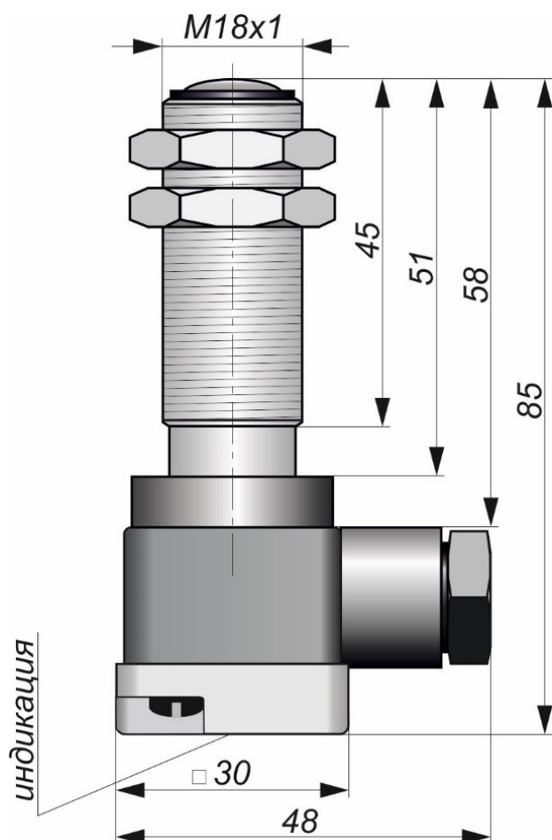
Габаритный чертеж
