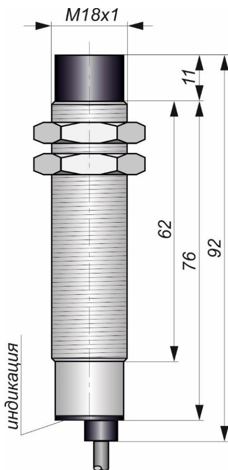
Габаритный чертеж
