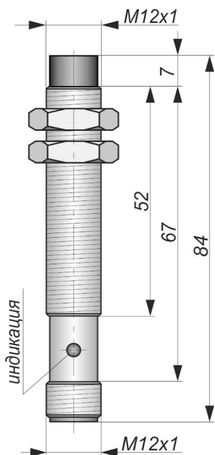
Габаритный чертеж
