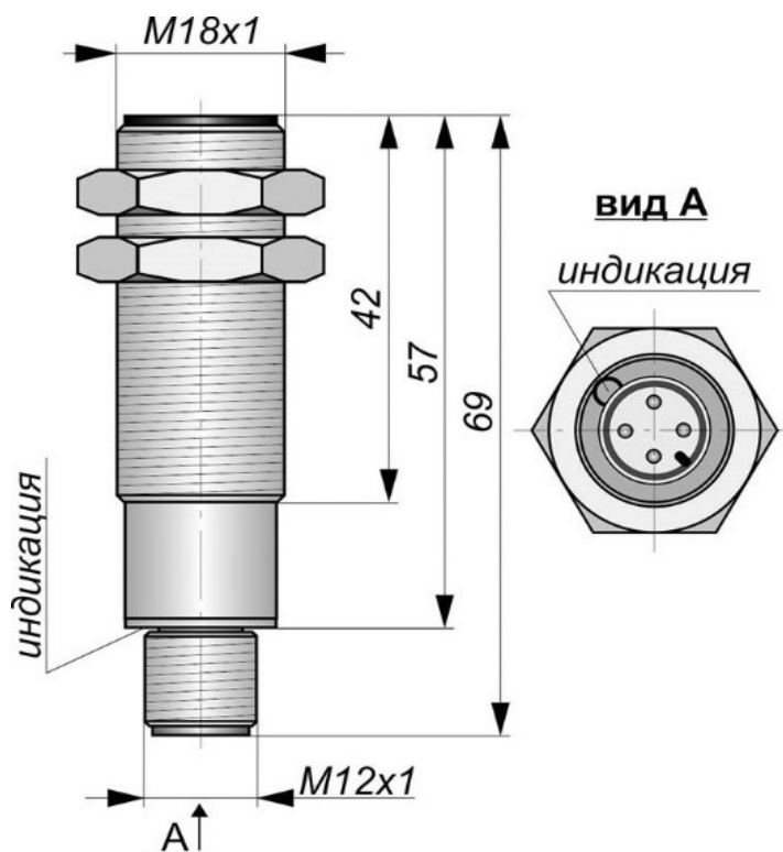
Габаритный чертеж
