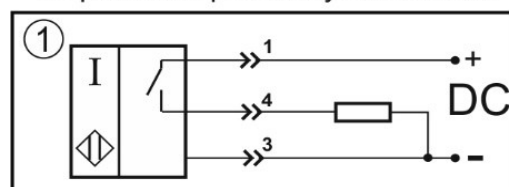
Цоколевка разъема
