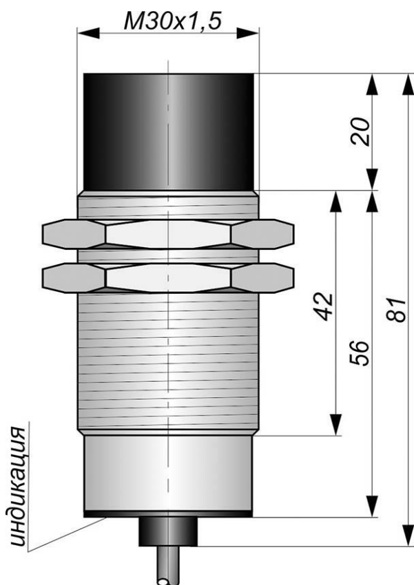
Габаритный чертеж
