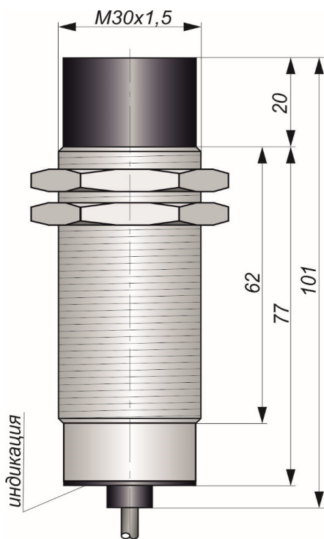
Габаритный чертеж
