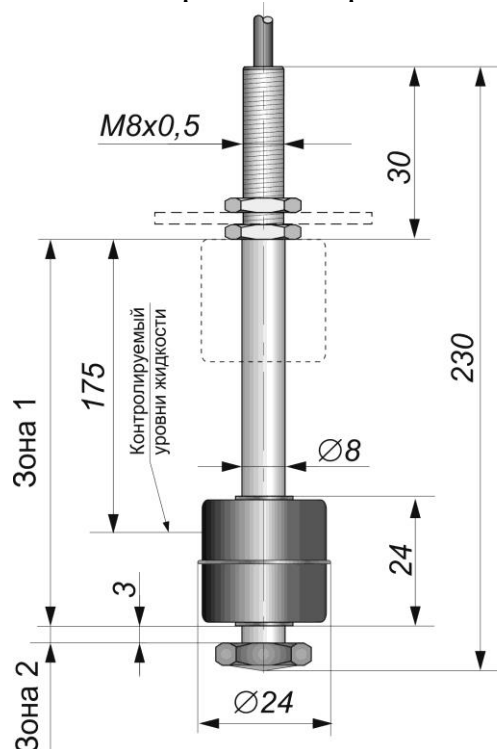
Габаритный чертеж
