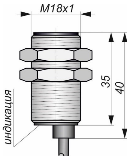
Габаритный чертеж
