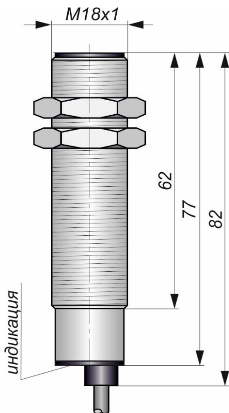
Габаритный чертеж
