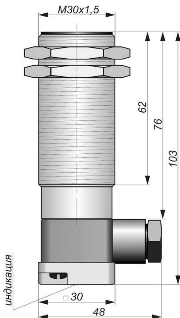
Габаритный чертеж
