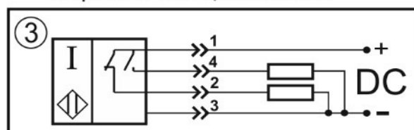
Переключающий контакт
