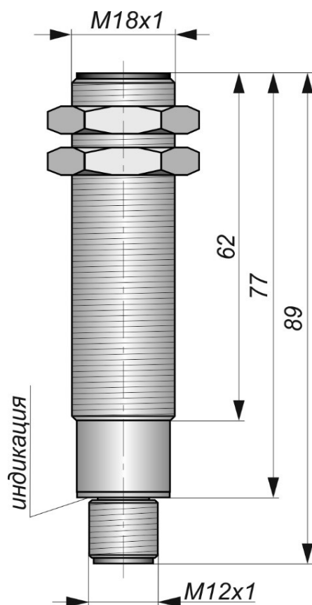
Габаритный чертеж
