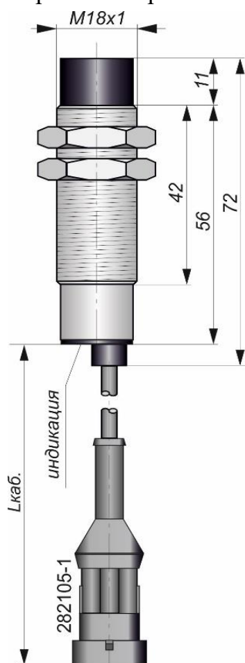
Габаритный чертеж
