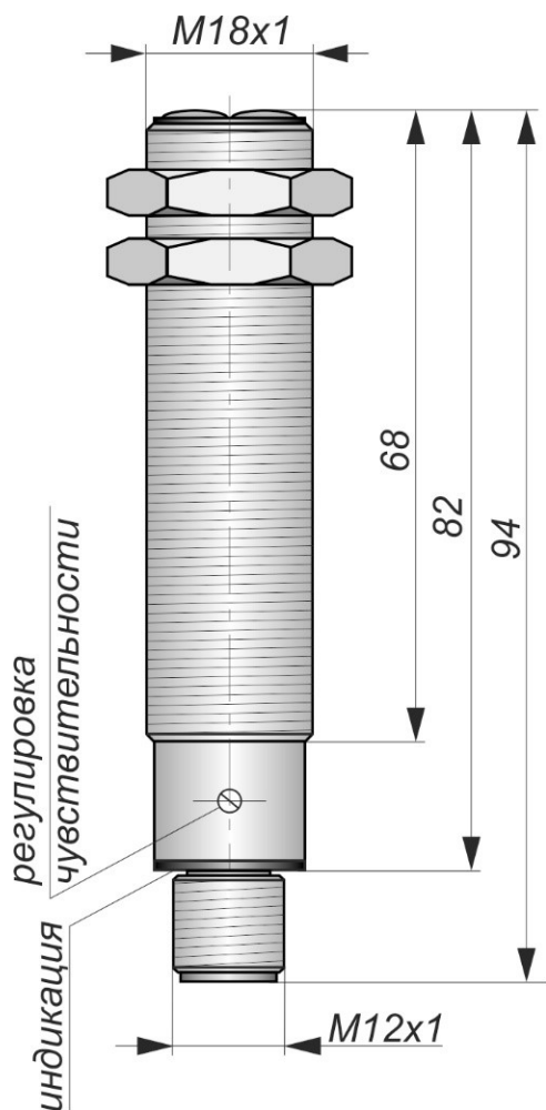
Габаритный чертеж
