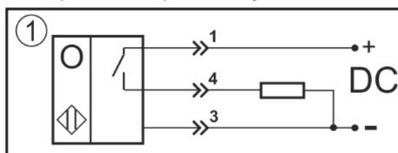
Цоколевка разъема
