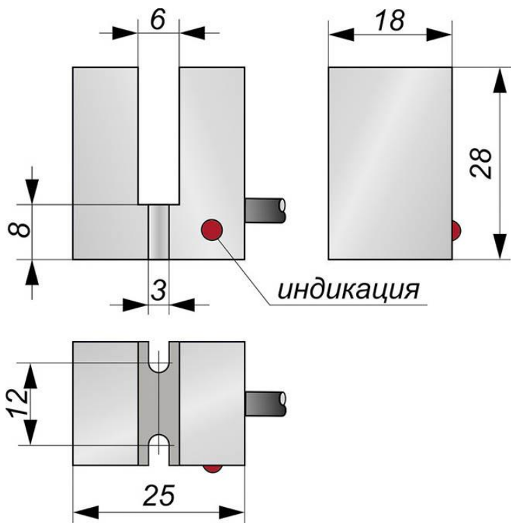
Габаритный чертеж
