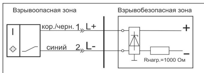
Схема соединения
