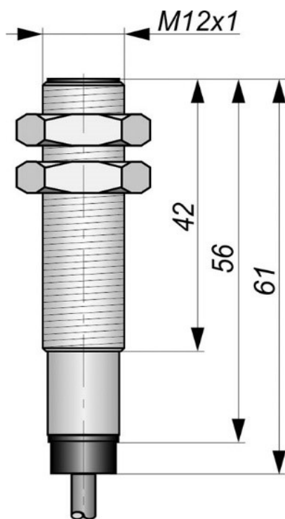
Габаритный чертеж
