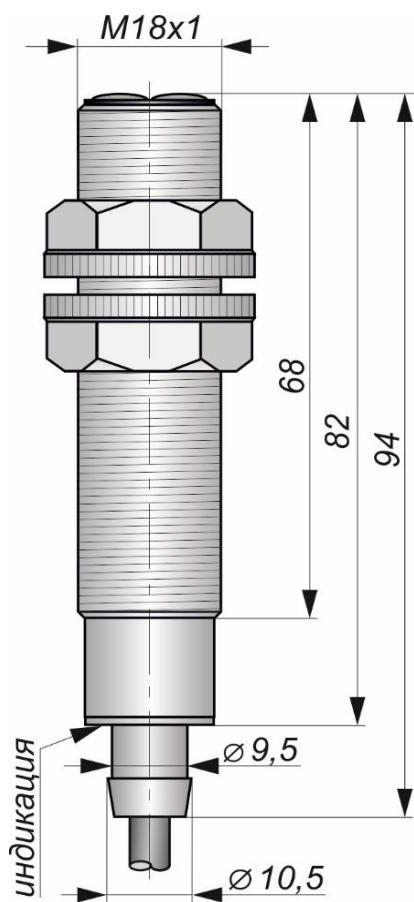
Габаритный чертеж
