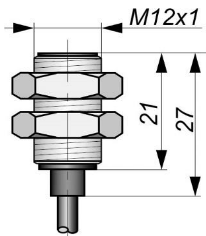
Габаритный чертеж
