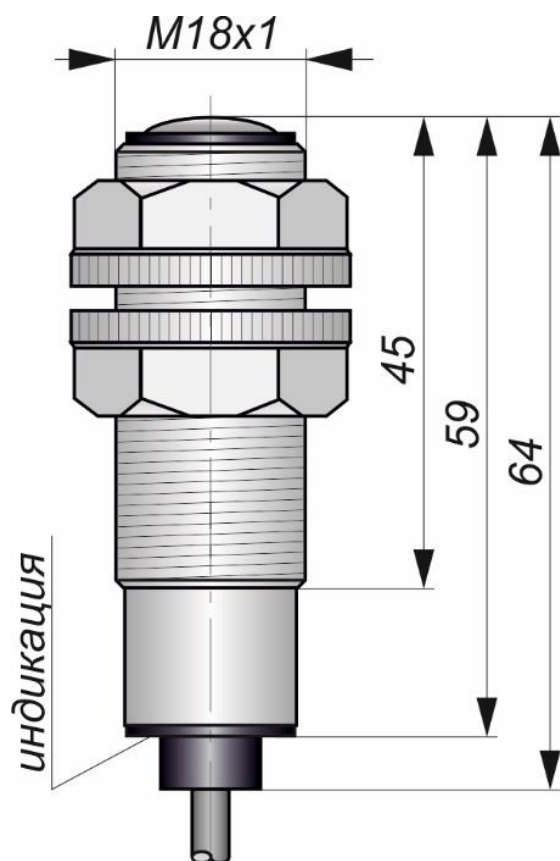
Габаритный чертеж
