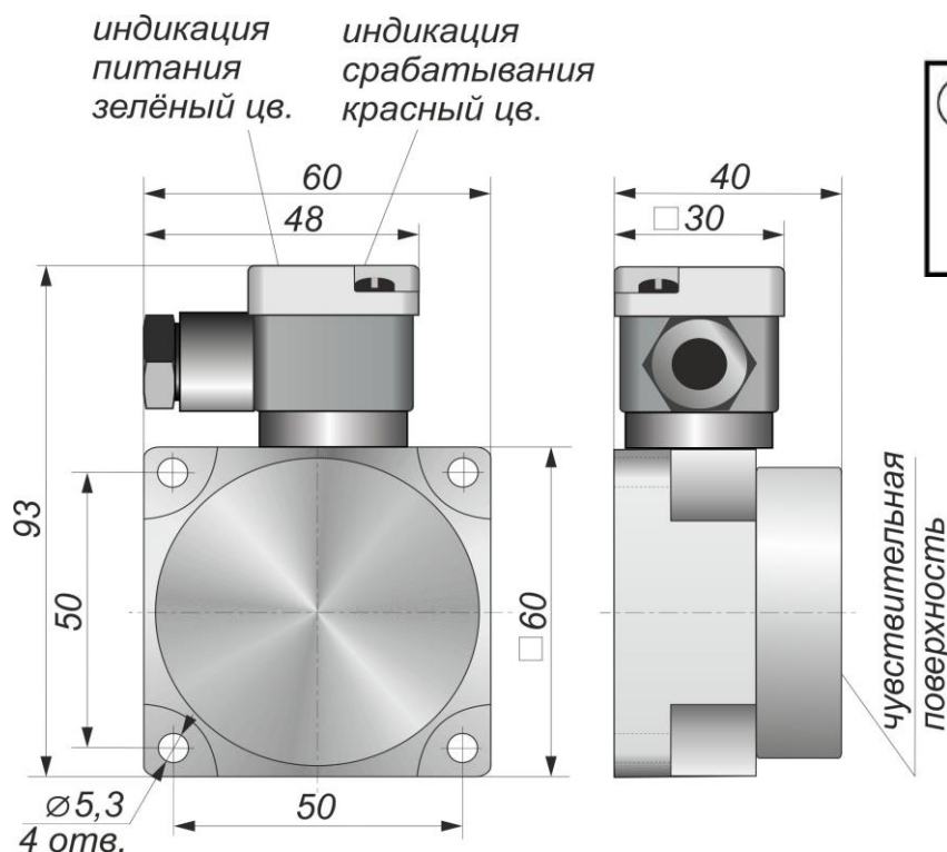
Габаритный чертеж
