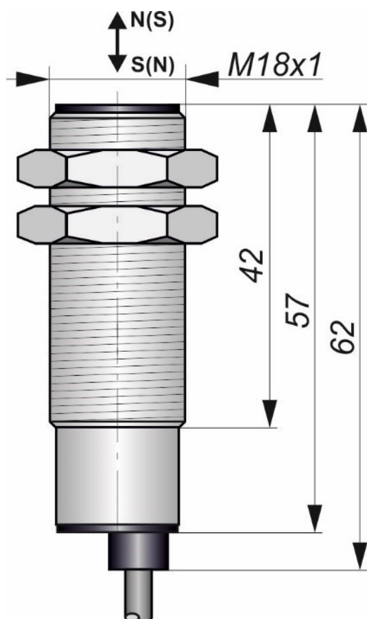
Габаритный чертеж
