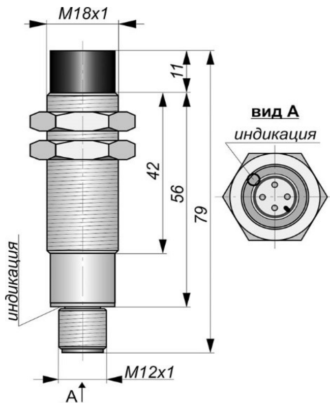
Габаритный чертеж
