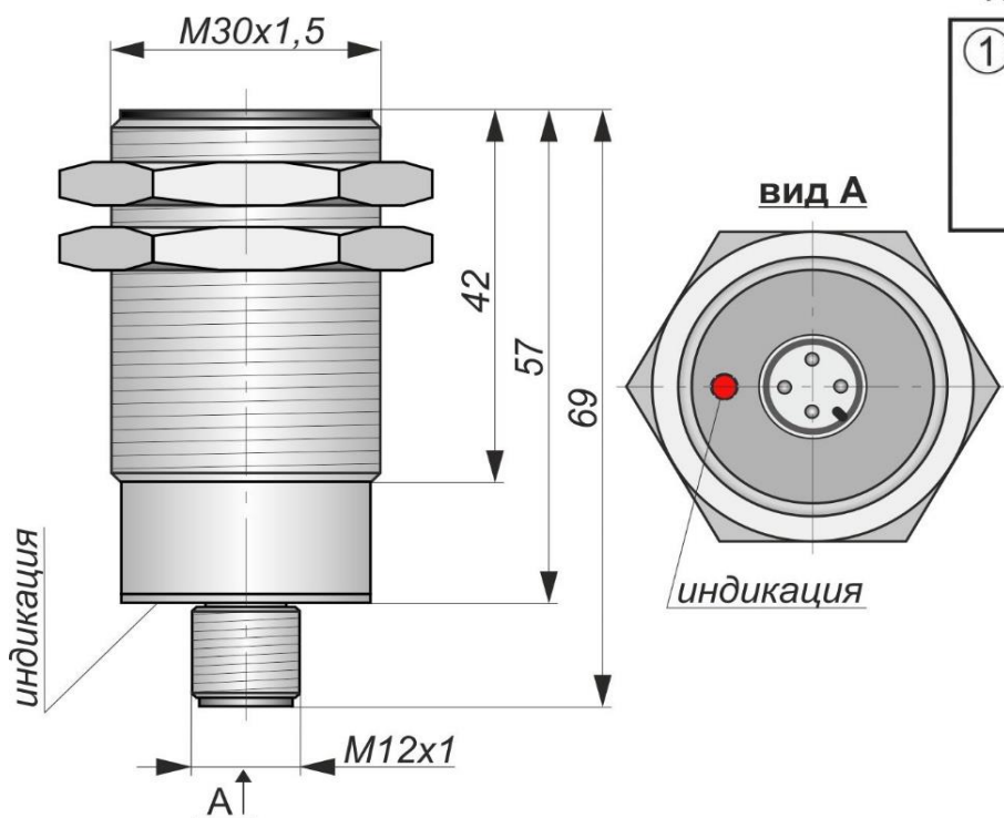
Габаритный чертеж
