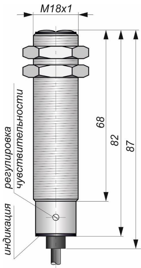
Габаритный чертеж
