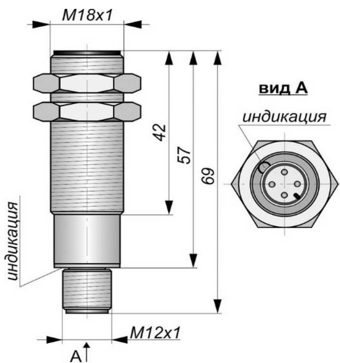
Габаритный чертеж
