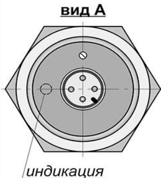
Цоколевка разъема
