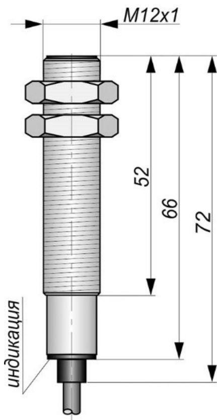
Габаритный чертеж
