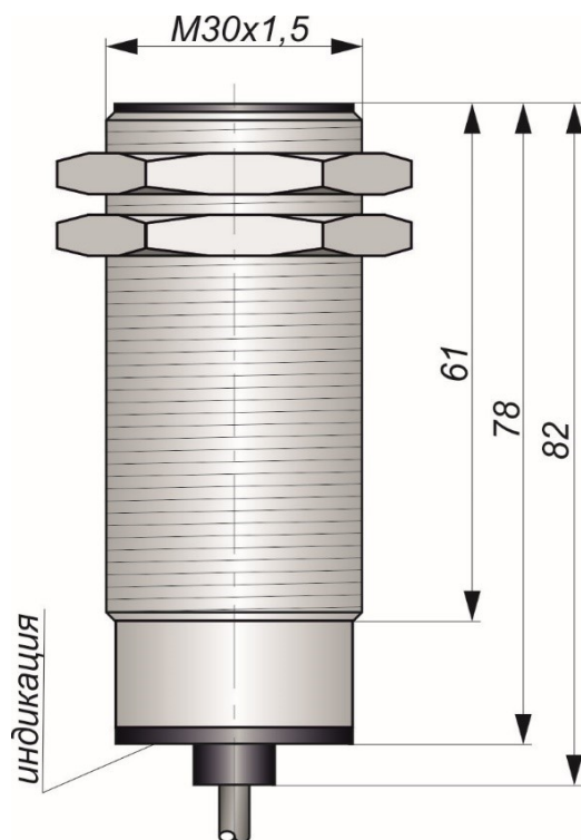
Габаритный чертеж
