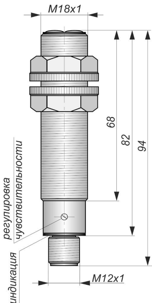
Габаритный чертеж
