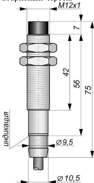
Габаритный чертеж
