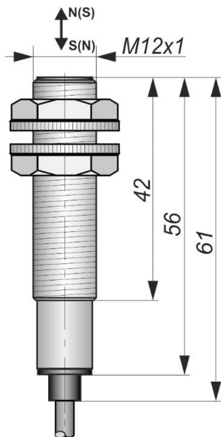
Габаритный чертеж
