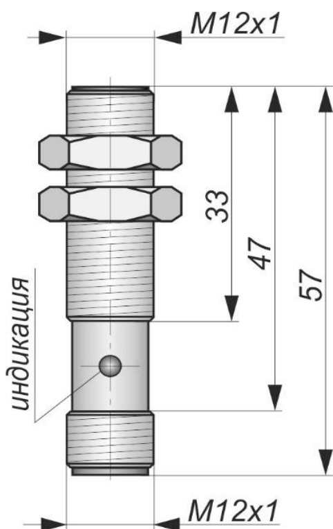
Габаритный чертеж
