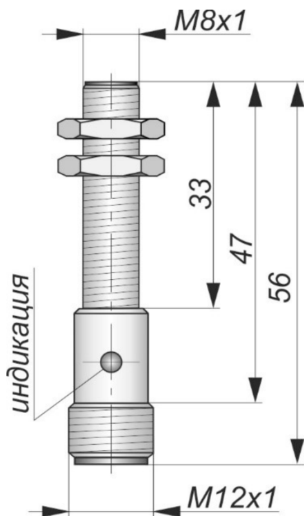
Габаритный чертеж
