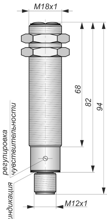
Габаритный чертеж
