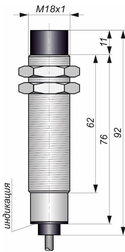
Габаритный чертеж
