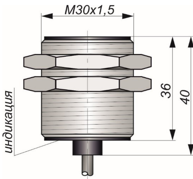
Габаритный чертеж
