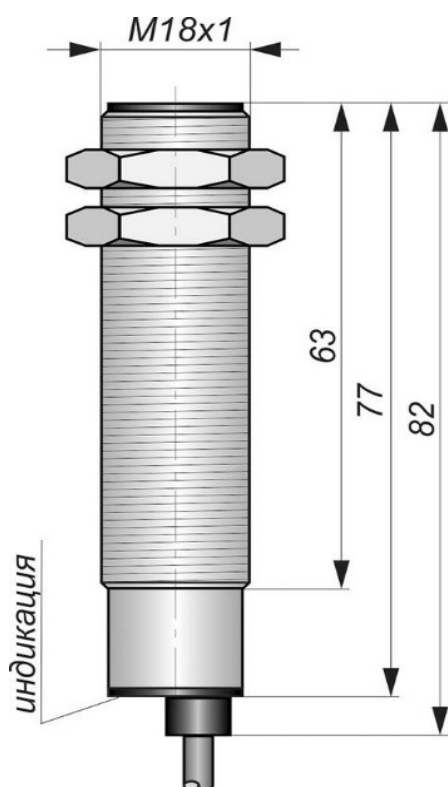
Габаритный чертеж
