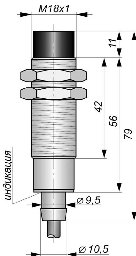
Габаритный чертеж
