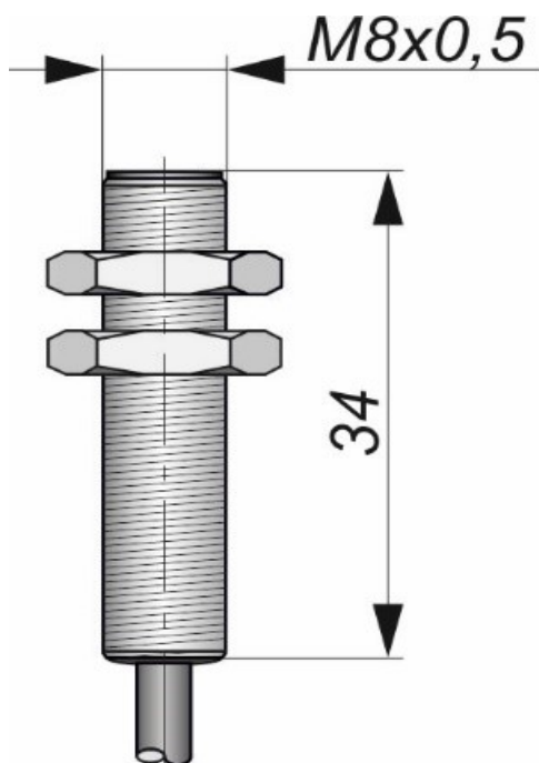
Габаритный чертеж
