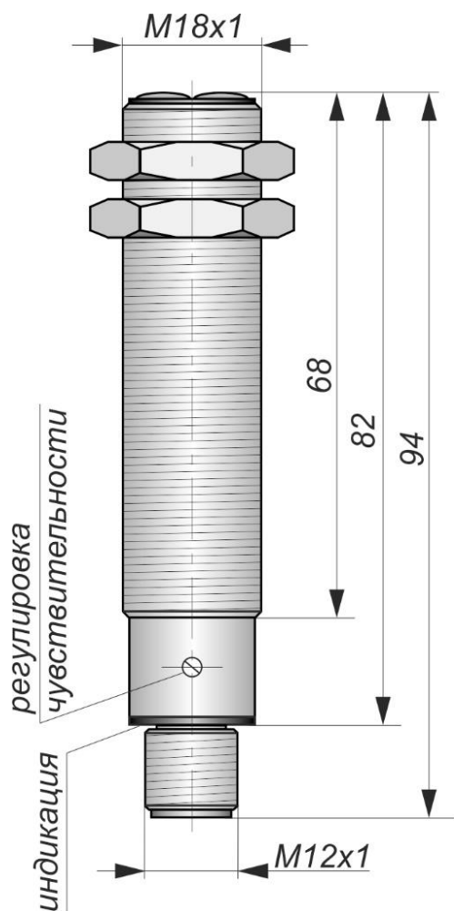
Габаритный чертеж
