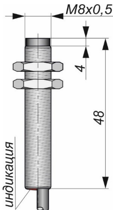
Габаритный чертеж
