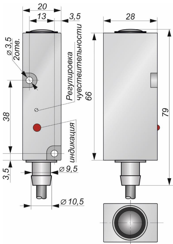
Габаритный чертеж
