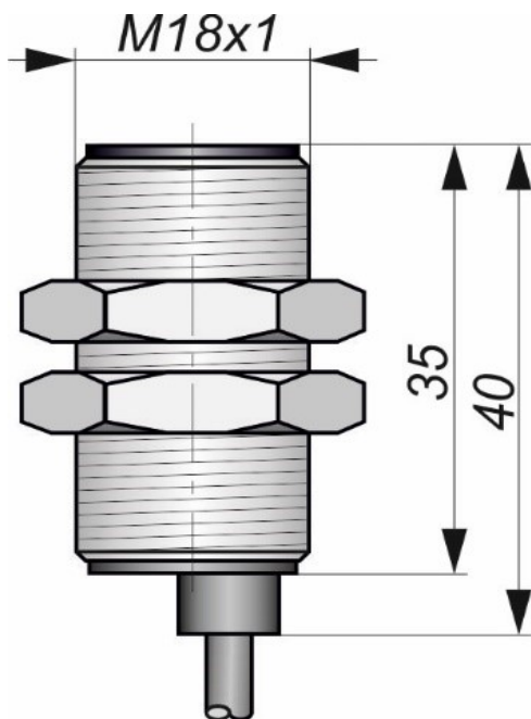
Габаритный чертеж
