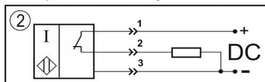
Цоколевка разъема
