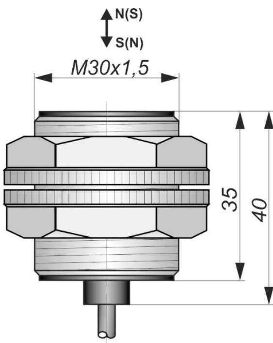
Габаритный чертеж
