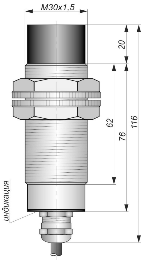
Габаритный чертеж
