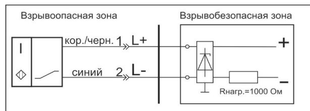
Схема соединения
