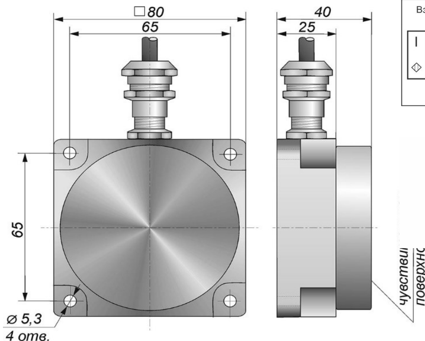
Габаритный чертеж
