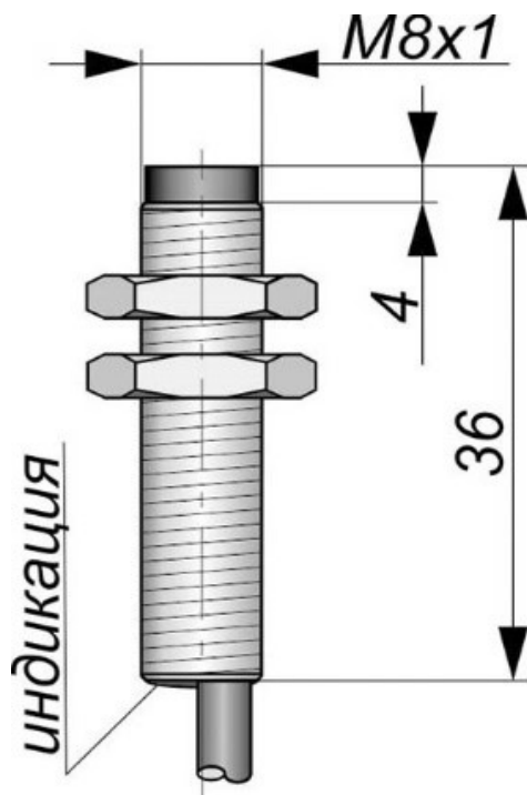
Габаритный чертеж
