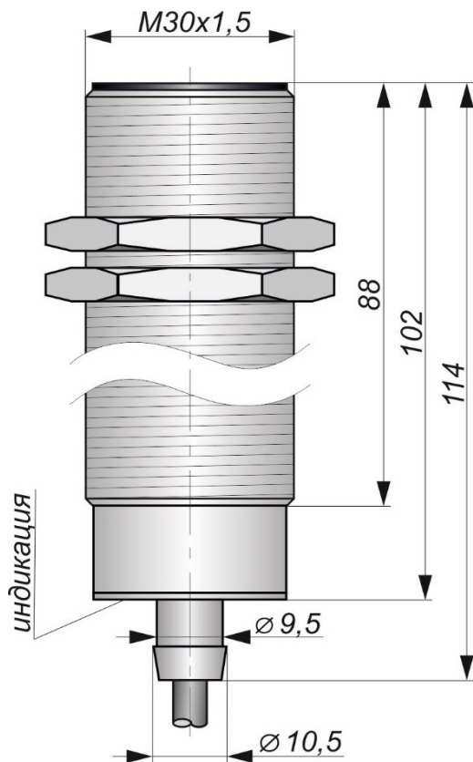
Габаритный чертеж
